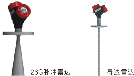
26G脉冲雷达
