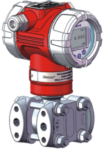
DP1300-DR微差压变送器
