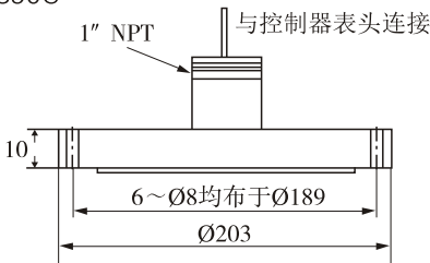
平板探头L890C
