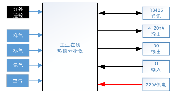
热值仪在应用系统中的接口示意图
