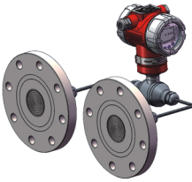
DP1300-YC远传差压变送器
